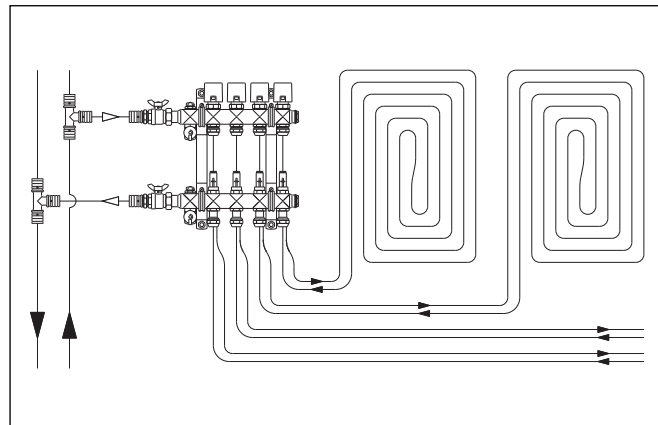
напольное отопление
