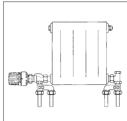
Напольное подсоединение с помощью h-элемента в 1- и 2-трубных системах
